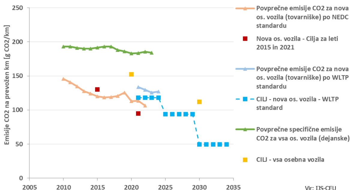
Slika 5: Povprečni izpusti CO 2 novih vozil s cilji za leto 2015 in 2021 po NEDC standardu, povprečni izpusti CO 2 novih vozil po WLTP standardu s cilji po WLTP standardu za obdobje od leta 2021 do leta 2034 ter povprečni izpusti CO 2 vseh vozil in cilji za leti 2020 in 2030 (Vir: ARSO, IJS-CEU)
