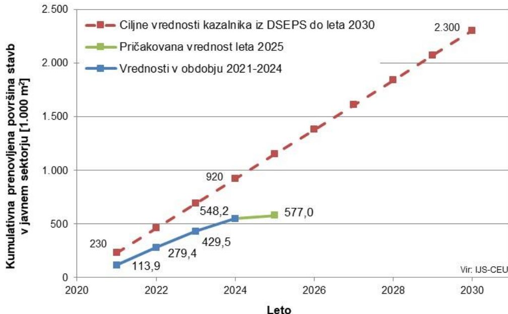
Slika 15: Kumulativna površina celovito energetske saniranih stavb v javnem sektorju v obdobju 2021–2024, pričakovana vrednost kazalnika leta 2025 39 ter njegove ciljne vrednosti do leta 2030 (Vir: IJS-CEU)
