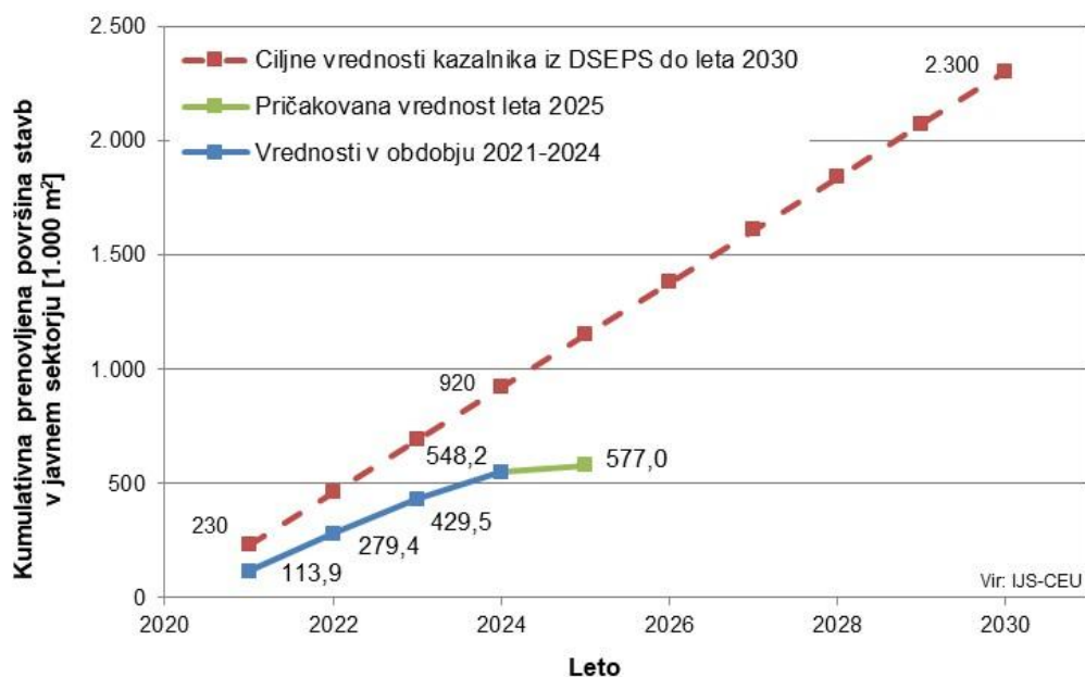
Slika 3: Kumulativna površina celovito energetsko saniranih stavb v javnem sektorju v obdobju 2021–2024, pričakovana vrednost kazalnika leta 2025 12 ter njegove ciljne vrednosti do leta 2030 (Vir: IJS-CEU)
