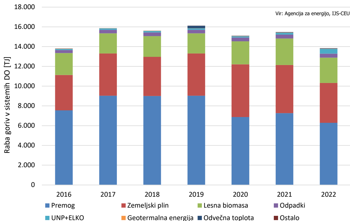
Slika 30: Struktura porabe goriv v vseh sistemih daljinskega ogrevanja v obdobju 2016–2022 (Vir: Agencija za energijo, IJS-CEU) Fuel consumption structure in all district heating systems in the period 2016–2022 (Source: Energy Agency, JSI-EEC)
