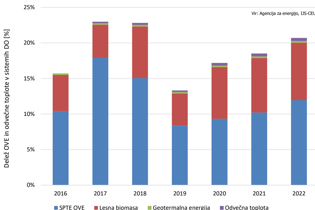
Slika 29: Struktura proizvodnje toplote iz OVE in odvečne toplote v vseh sistemih daljinskega ogrevanja v obdobju 2016–2022 (Vir: Agencija za energijo, IJS-CEU)
