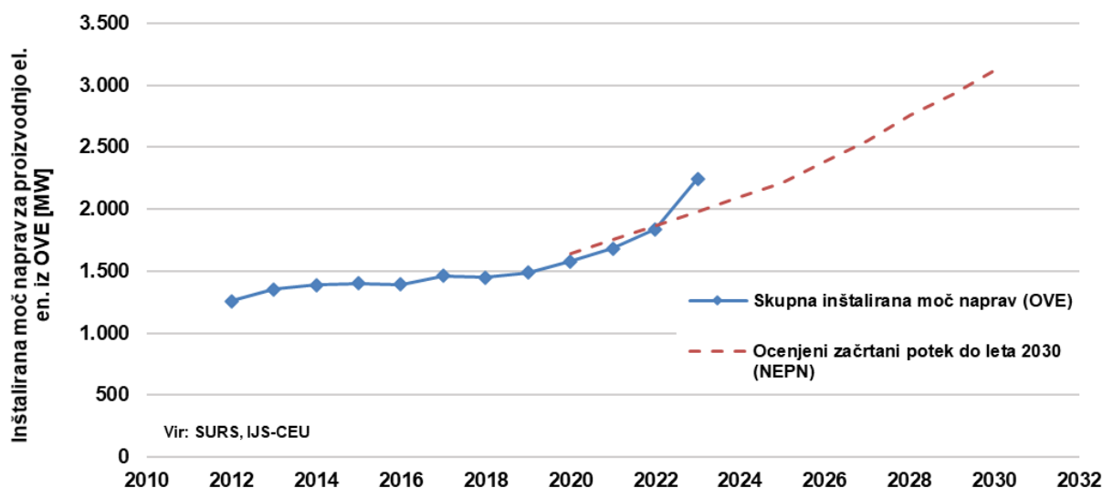
Slika 18: Inštalirana moč naprav za proizvodnjo električne energije iz obnovljivih virov energije v obdobju 2012–2023 in indikativna ciljna trajektorija do leta 2030 (brez vpoštevanja črpalnih hidroelektrarn) (Vir: SURS, IJS-CEU) Installed capacity of the systems for the production of electricity from RES in the period 2012–2023 and its target values up to 2030 (pure pumped hydro storage plants are not included) (Source: Republic of Slovenia Statistical Office, JSI-EEC)
