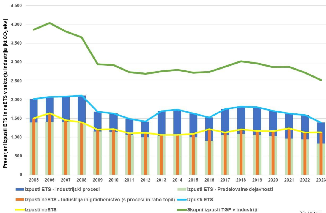
Slika 3: Izpusti EU-ETS in neETS v sektorju industrija, razdeljeni na predelovalne dejavnosti in industrijske procese, v obdobju 2005–2023 (Vir: IJS-CEU)
