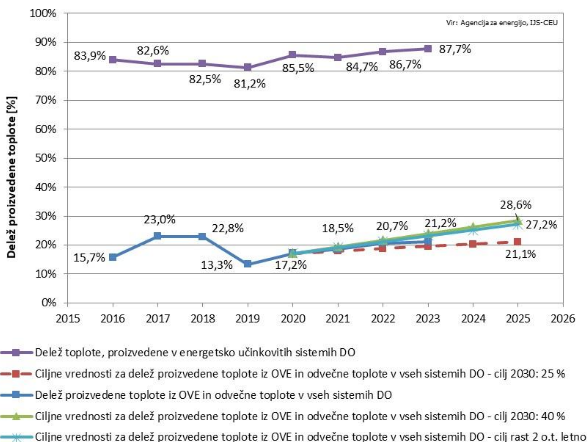
Slika 6: Delež toplote, proizvedene v energetske učinkovitih sistemih daljinskega ogrevanja (DO) ter delež proizvedene toplote iz OVE in odvečne toplote v vseh sistemih DO in njegove indikativne ciljne vrednosti iz NEPN 2024 (Vir: Agencija za energijo, IJS-CEU)
